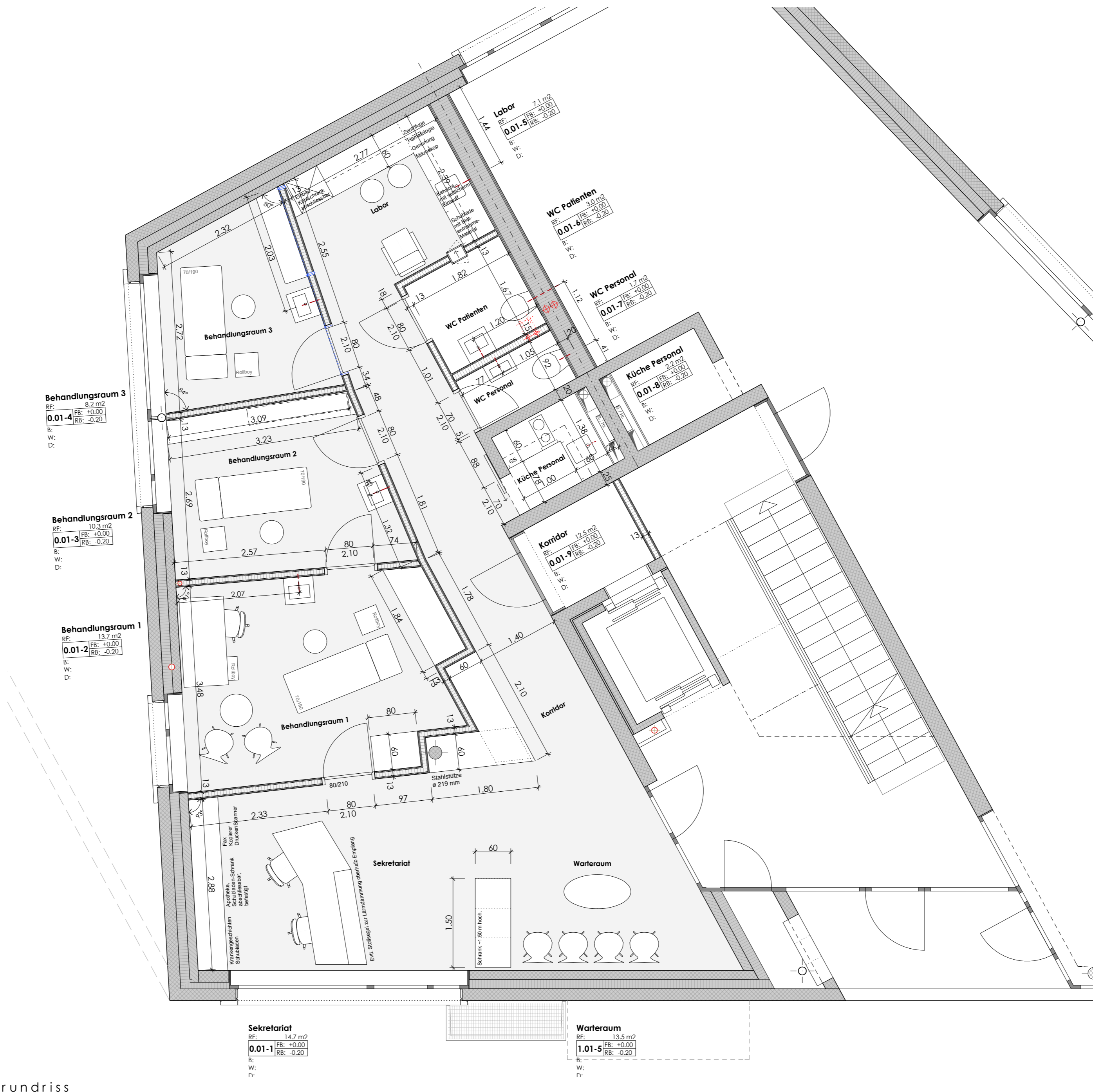
Grundriss
